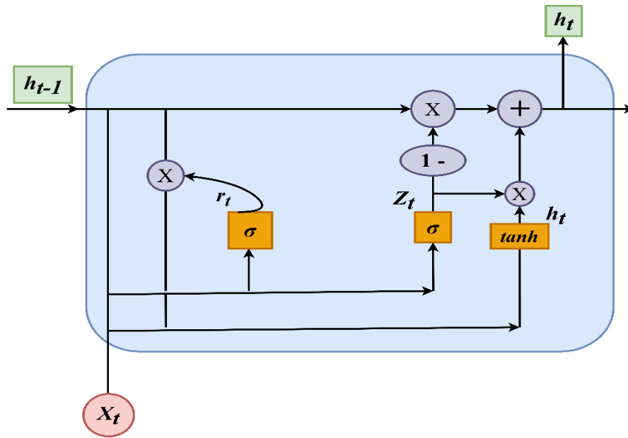
Fig. 4. GRU architecture
